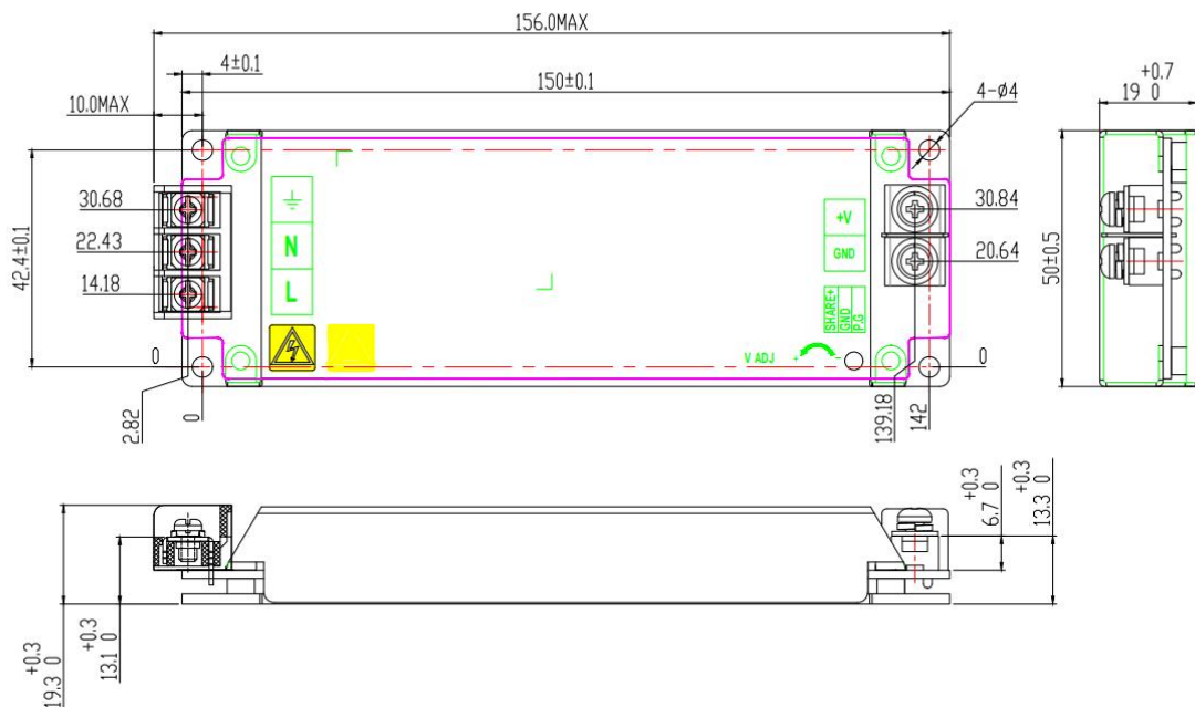
输入、输出端子定义及安装扭力
